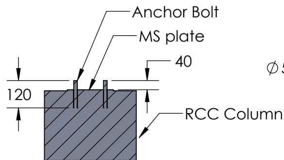
SECTION A-A SCALE 1 : 16
